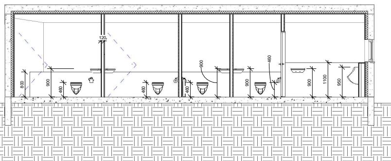
Snið B-B mkv: 1 : 50
