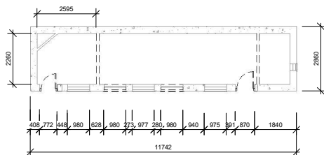
Grunnmynd fyrir, Mkv. 1:100
