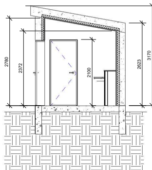
Snið A-A mkv: 1 : 50
