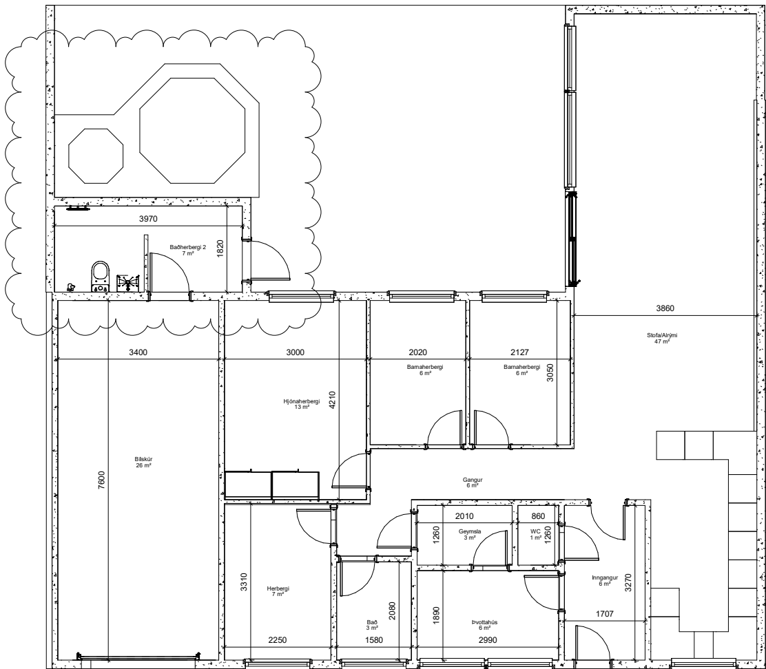
1 Grunnmynd - 1. hæð 1 : 50
