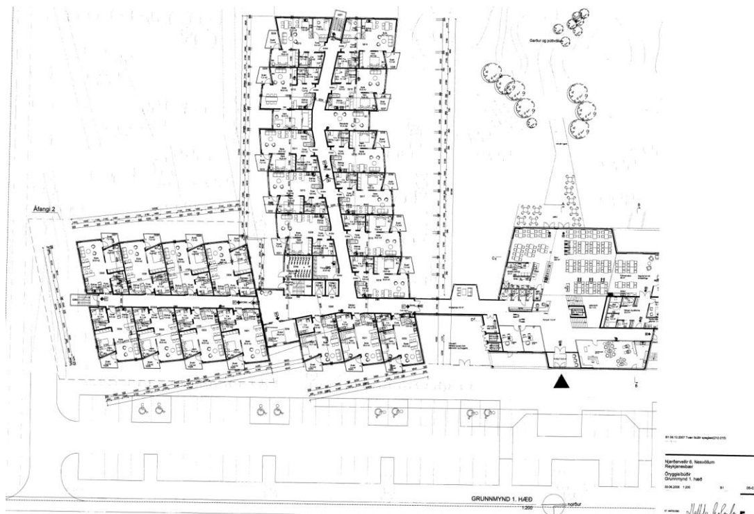
Mynd 10. Hluti grunnmynda 1. hæðar – inngangur og sameiginleg umferðarrými.
