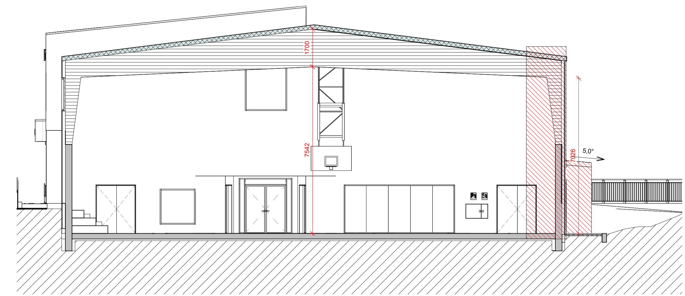
2 S-128 SNIÐ ÍÞRÓTTAHÚS - LOFTHÆÐ OG STÆKKUN 1 : 100
