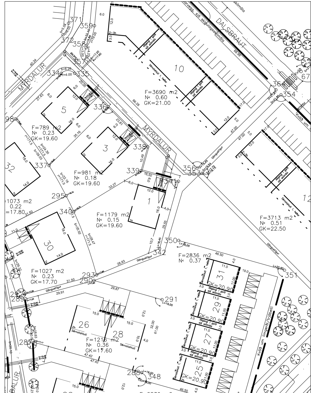
Afstöðumynd Mvk. 1:500
