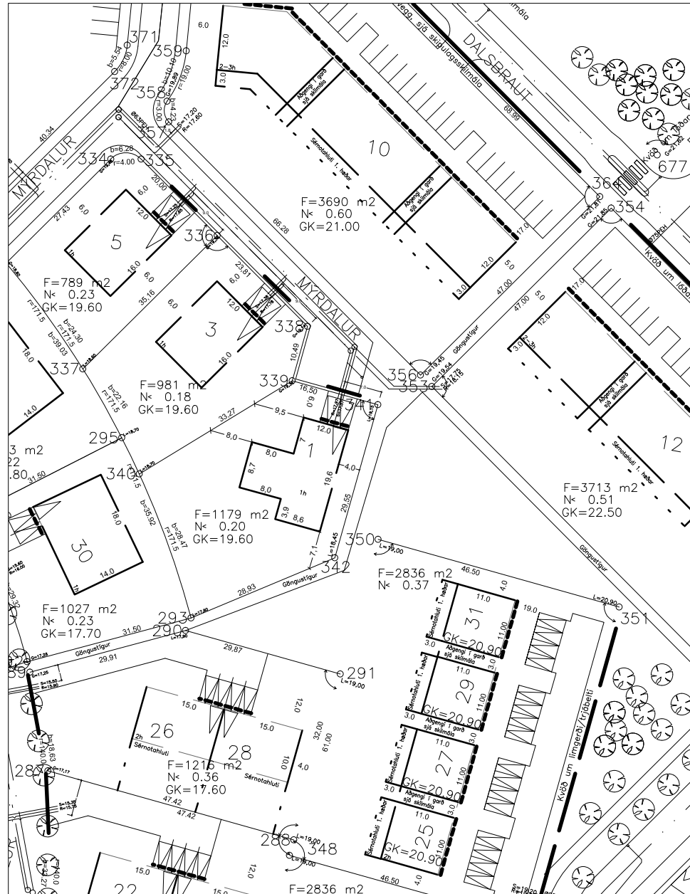
Afstöðumynd Mvk. 1:500
