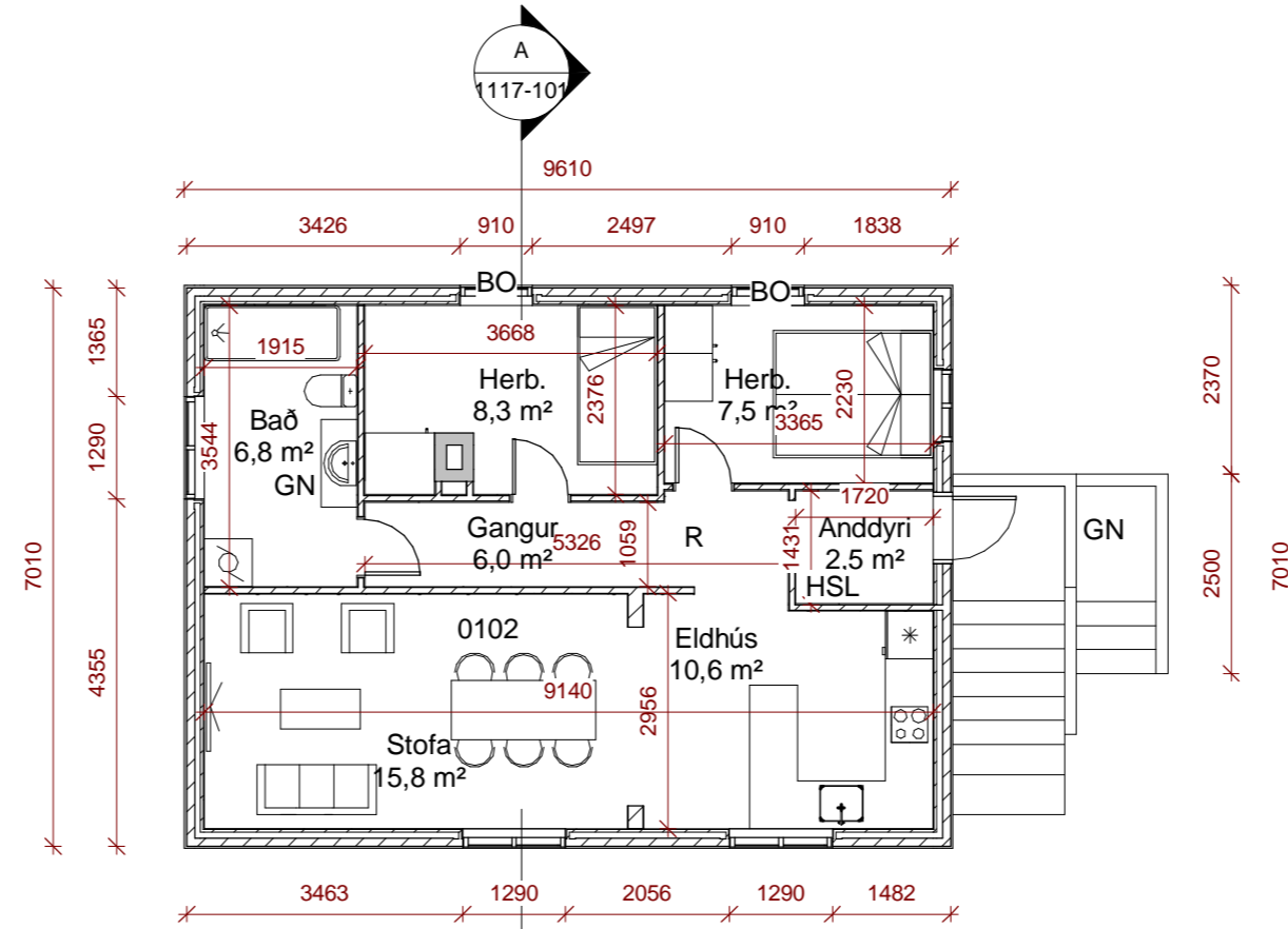
Grunnmynd 2. hæð 1 : 100
