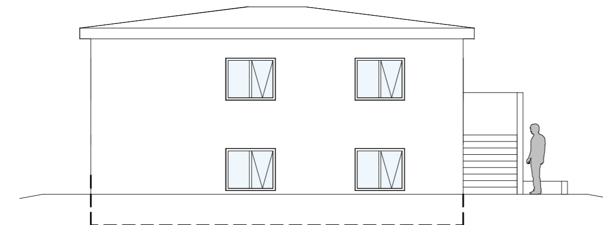
Austur 1 : 100
