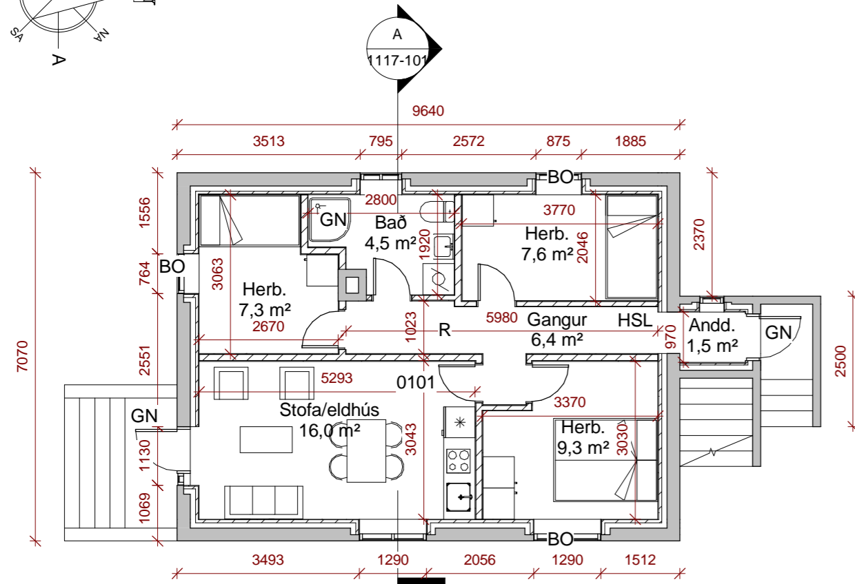
Grunnmynd 1. hæð 1 : 100
