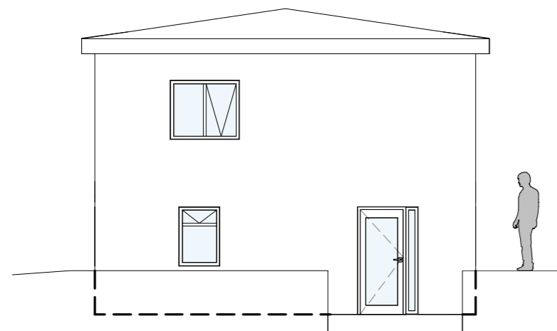
Suður 1 : 100
