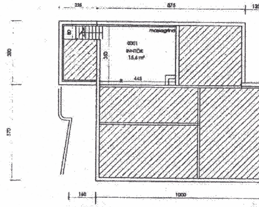
GRUNNMYND KJALLARA
