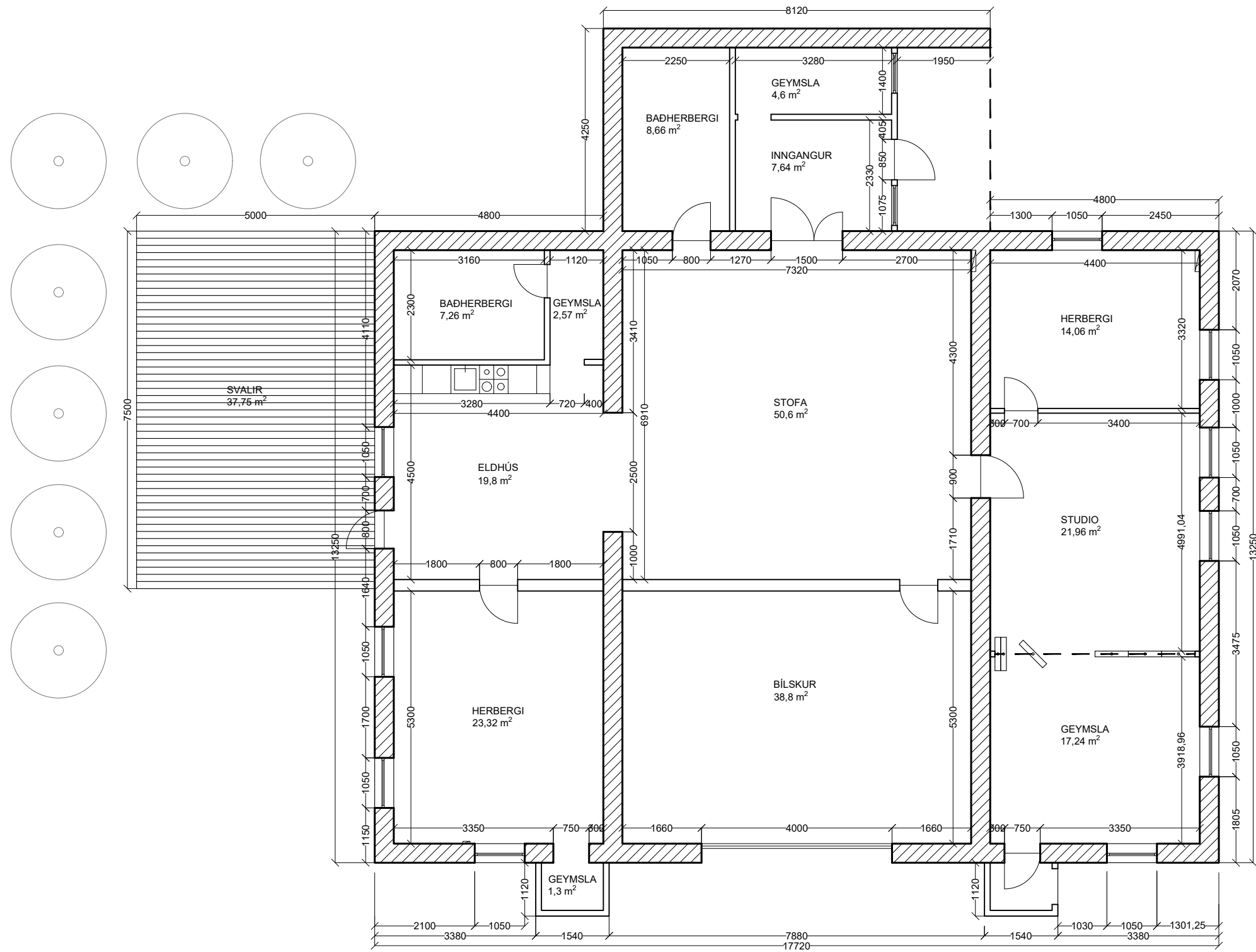
GRUNNMYND 1. HÆÐ - FRAMTÍÐARPLAN Mælikvarði 1:100
