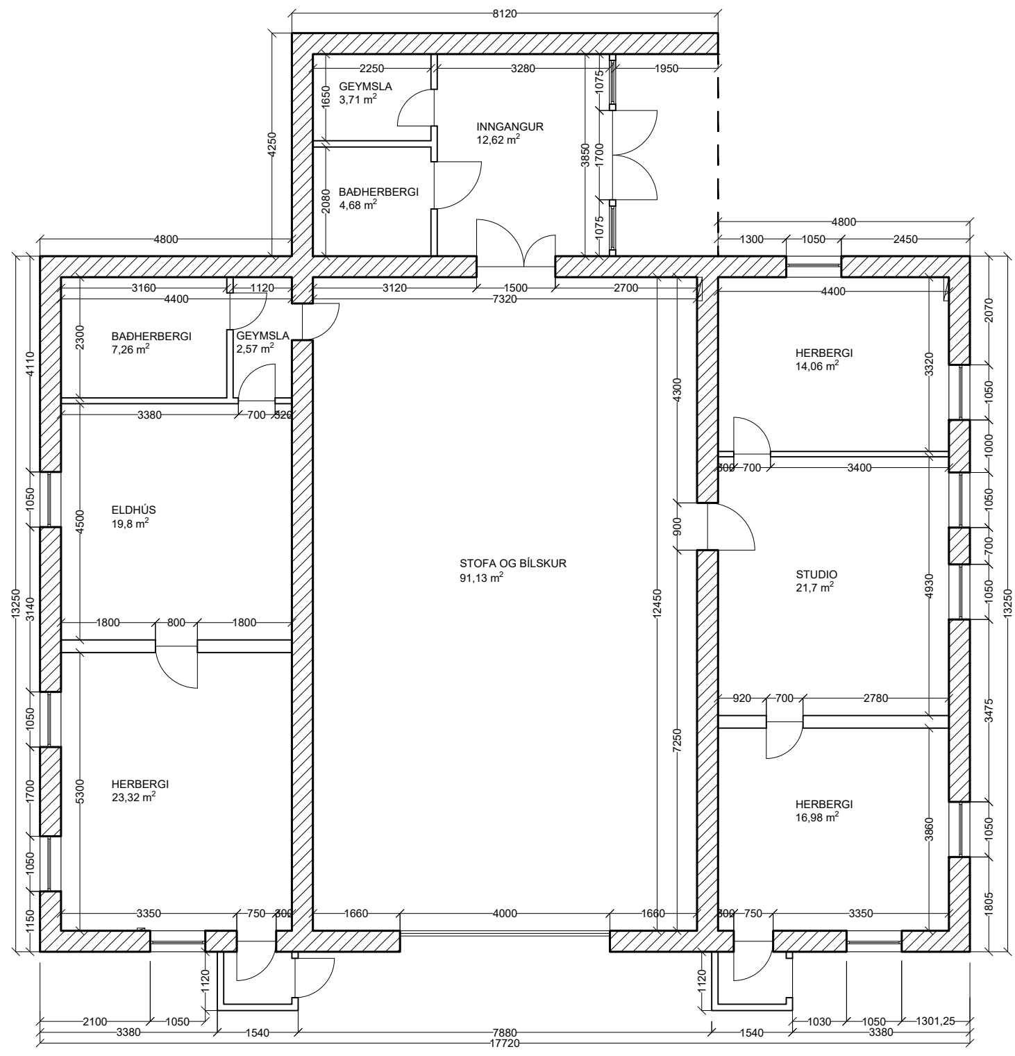
GRUNNMYND 1. HÆÐ - NÚVERANDI ÁSTAND Mælikvarði 1:100
