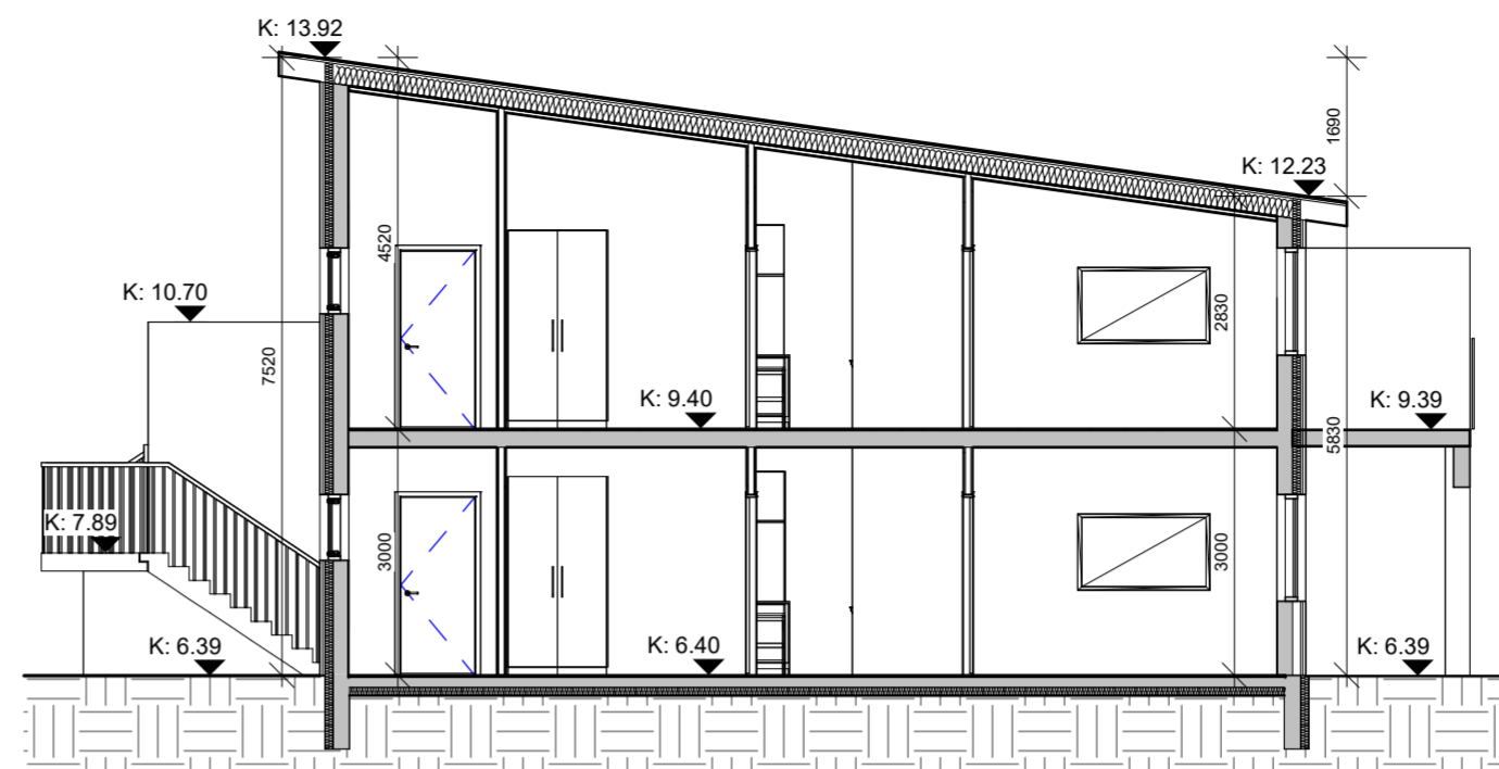
Snið 1:100
