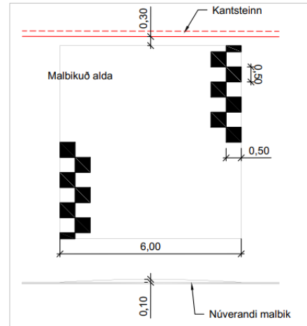
MYND 3 Til vinstri: Breytt rúnnuð hraðahindrun (Mynd frá Vejregler, 2014, bls. 45). Til hægri: Malbikuð rúnnuð upphækkun (Hönnun: EFLA).
