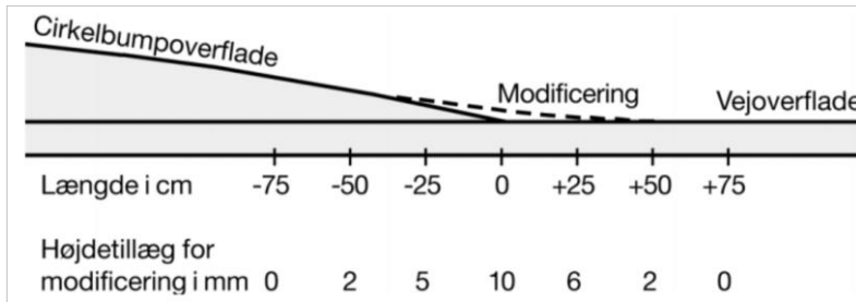
MYND 3 Til vinstri: Breytt rúnnuð hraðahindrun (Mynd frá Vejregler, 2014, bls. 45). Til hægri: Malbikuð rúnnuð upphækkun (Hönnun: EFLA).
