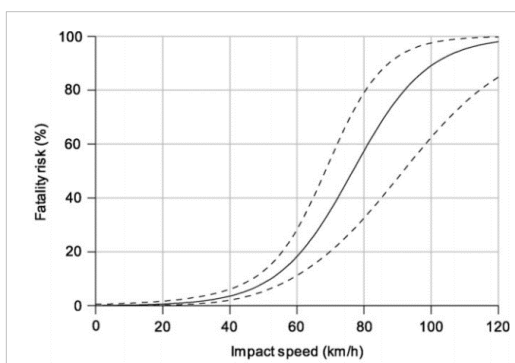
MYND 2 Til vinstri: Líkurnar á dauðfalli hjá fullorðnum fótgangandi sem fall af hraða ökutækis við áreksturinn. Strikalínurnar sýna 95% vikmörk. Til hægri: Samband á milli alvarleika slysa á gangandi vegfarendur sem verða fyrir ökutæki, aldur þeirra og hraða ökutækisins.
