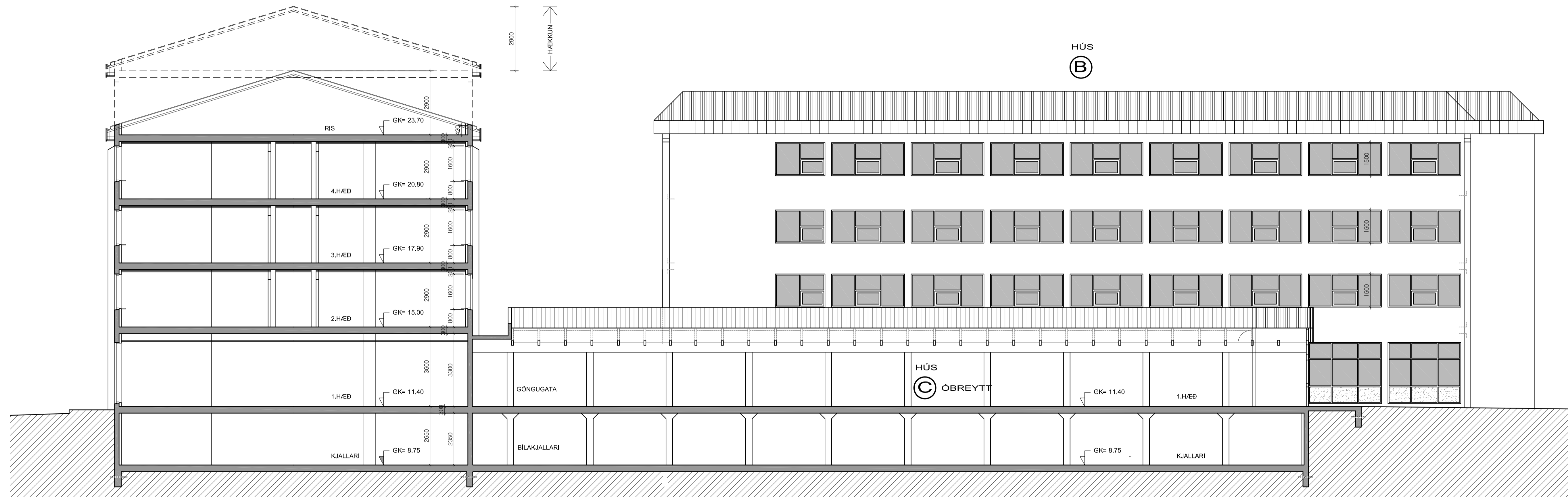
SNID / ÚTLIT C - C
