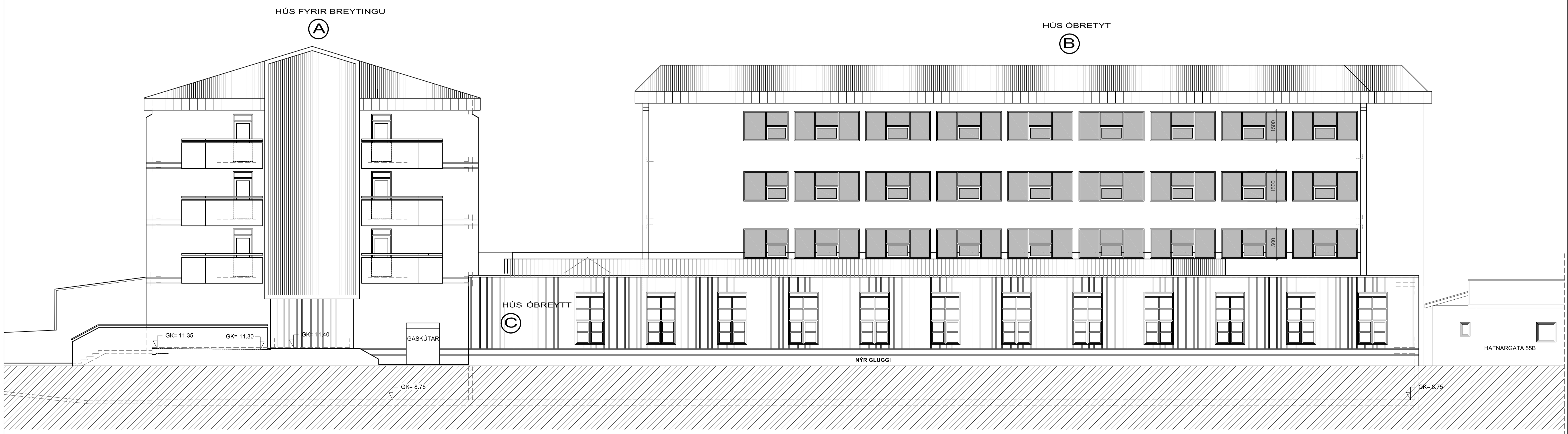
ÚTLIT AUSTUR / ÁSÝND B - B
