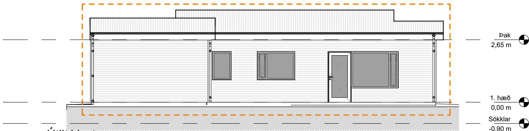
Útlit Vestur Mkv: 1:100
