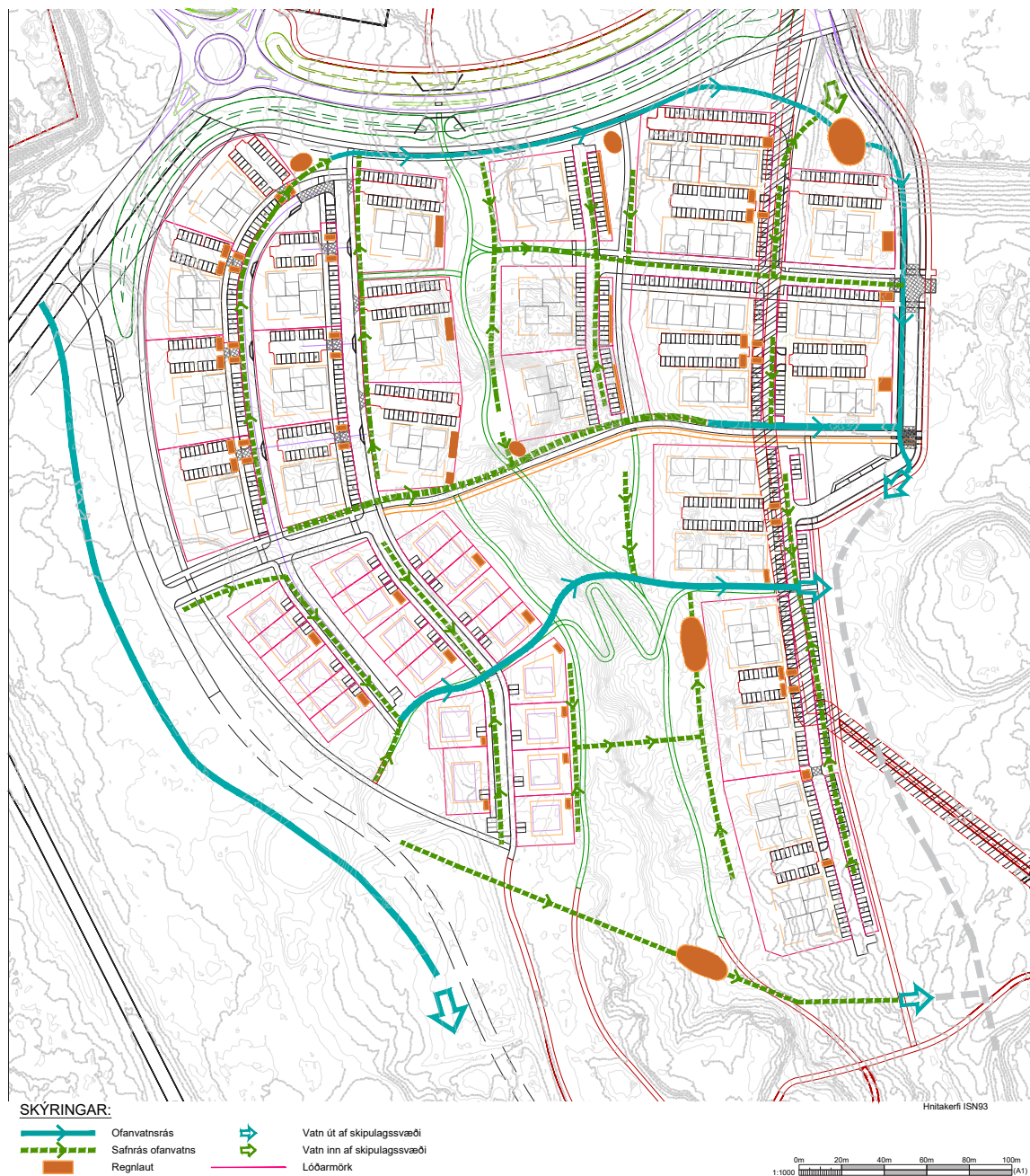
Mynd 15. Skýringarmynd Leiðbeinandi staðsetning ofanvatnsrása og regnlauta
