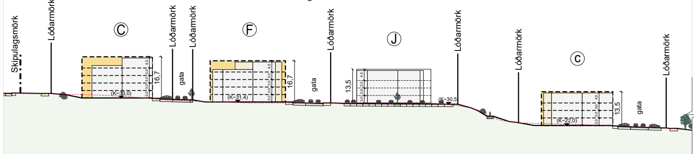
Sneiðing C-C
