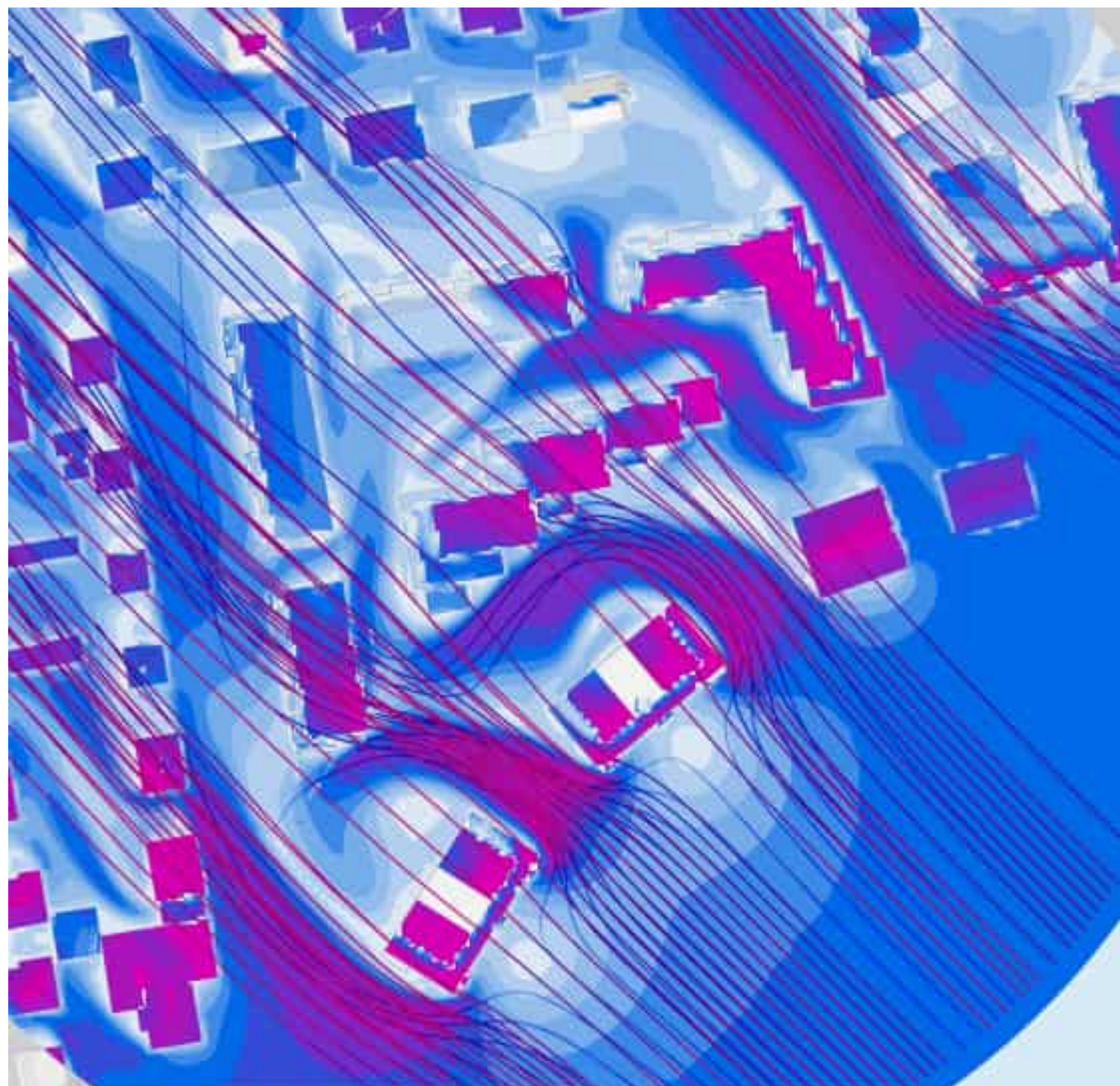
vindmæling, suðausturátt (10m/sek)
