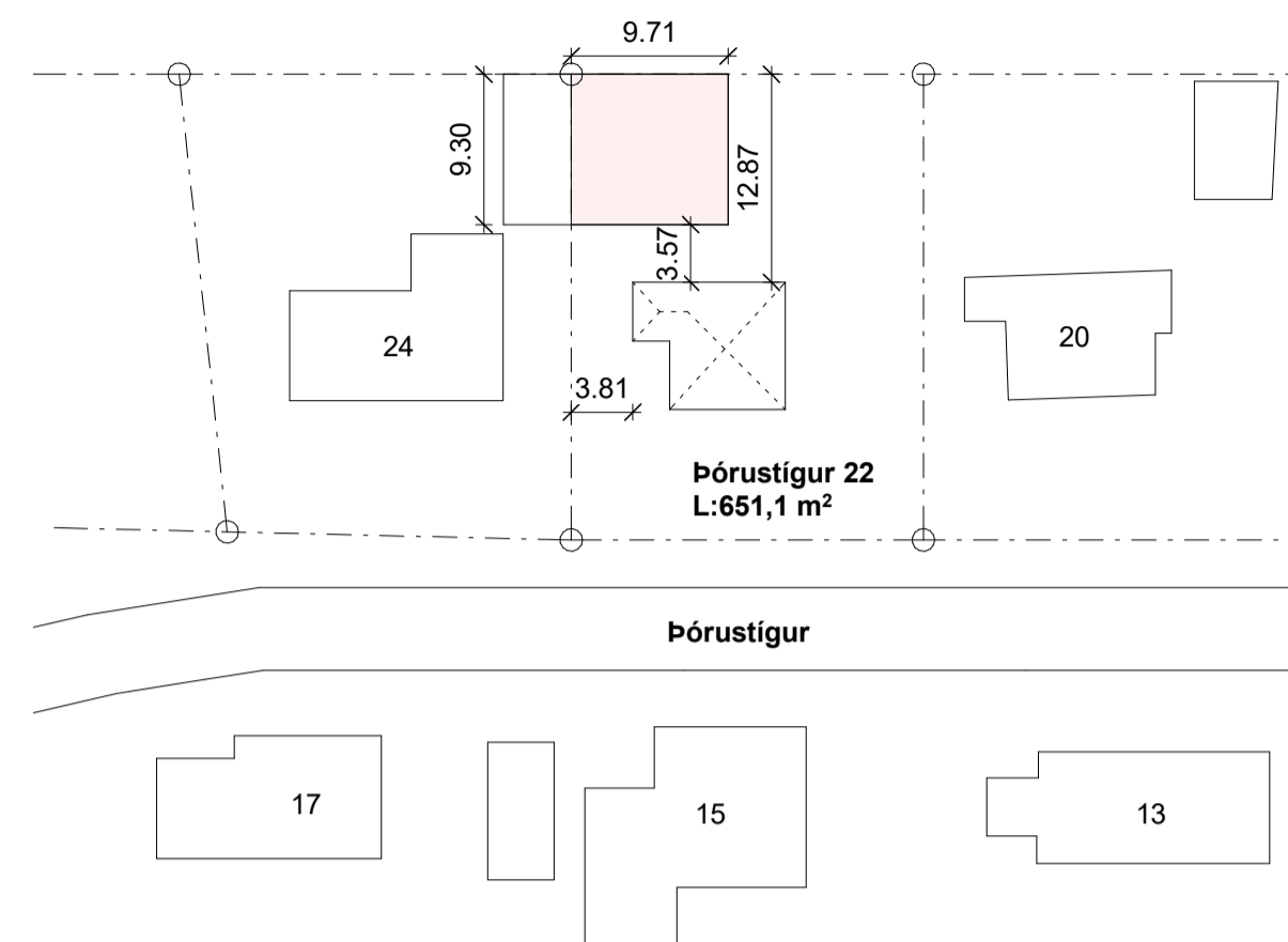
Afstöðumynd, Mkv.1:500
