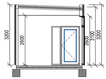
Snið A-A Mkv = 1:100
